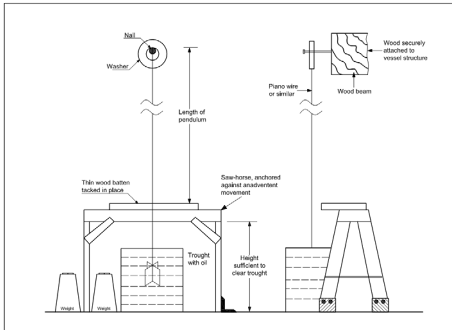
Fig. 1.3 Pendulum
