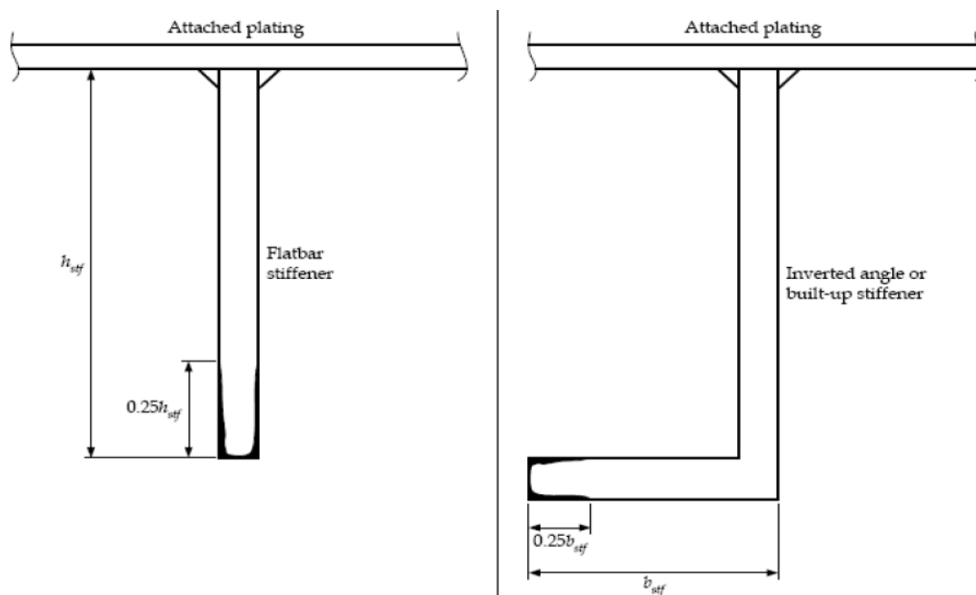
Fig. 1.2 Edge corrosion
